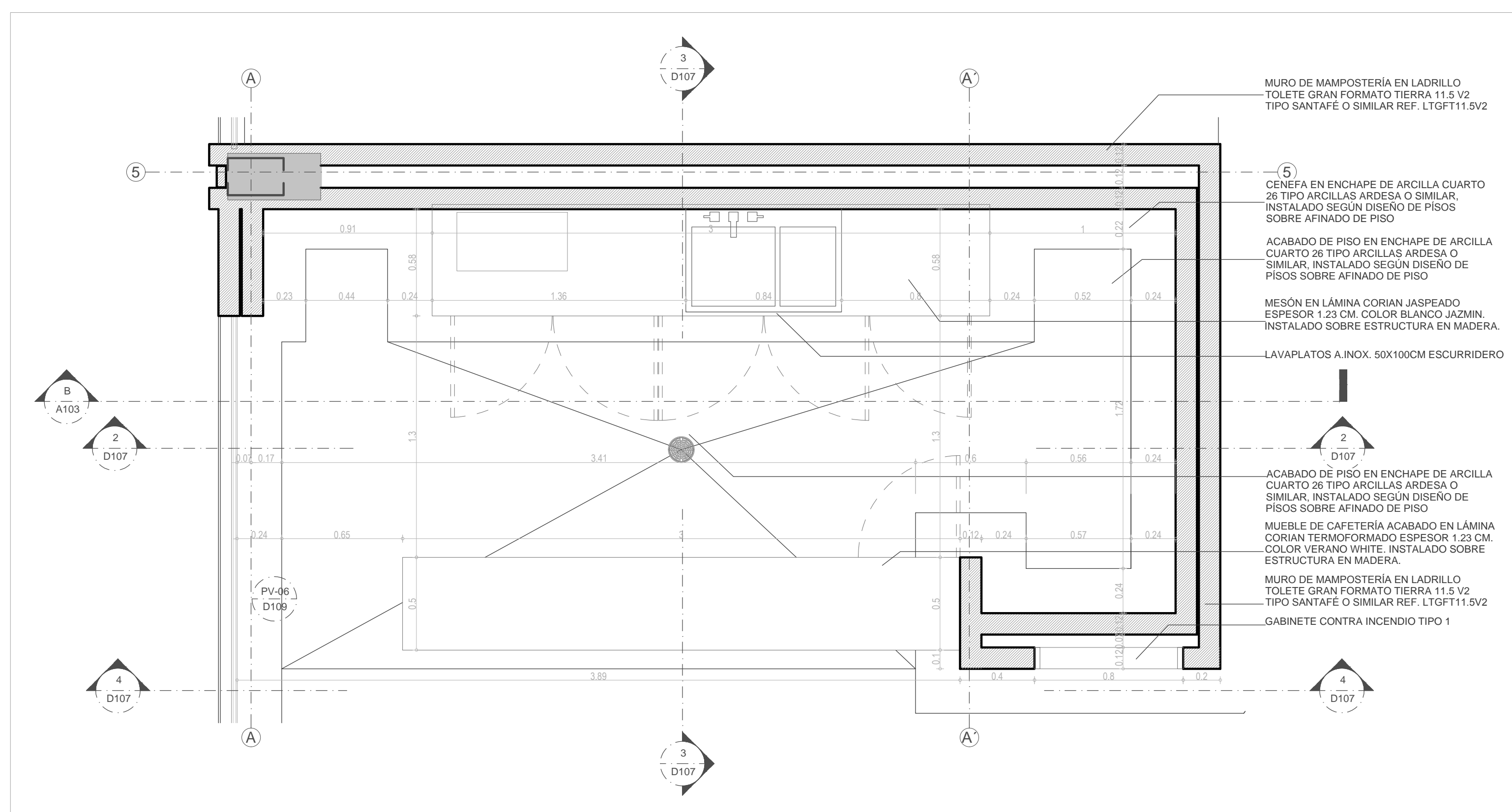
PLANTA DETALLE COCINA
