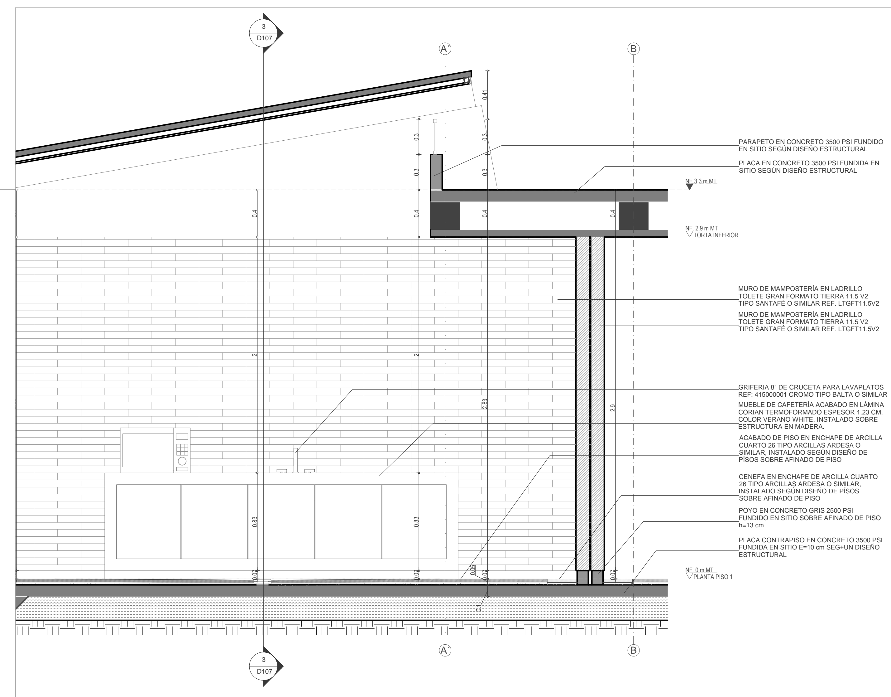
CORTE 1 COCINA
