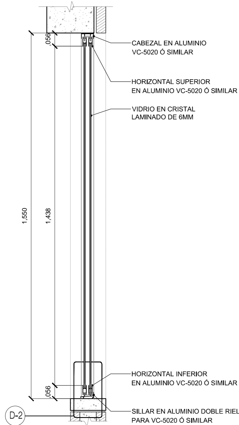
SECCIÓN VENTANA V-140
