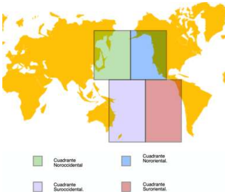
Gráfico 2. Cuadrantes del Océano Pacífico
